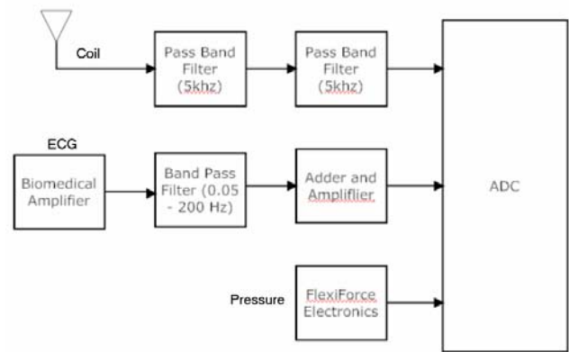
Fig. 1 Analog subsystem.
